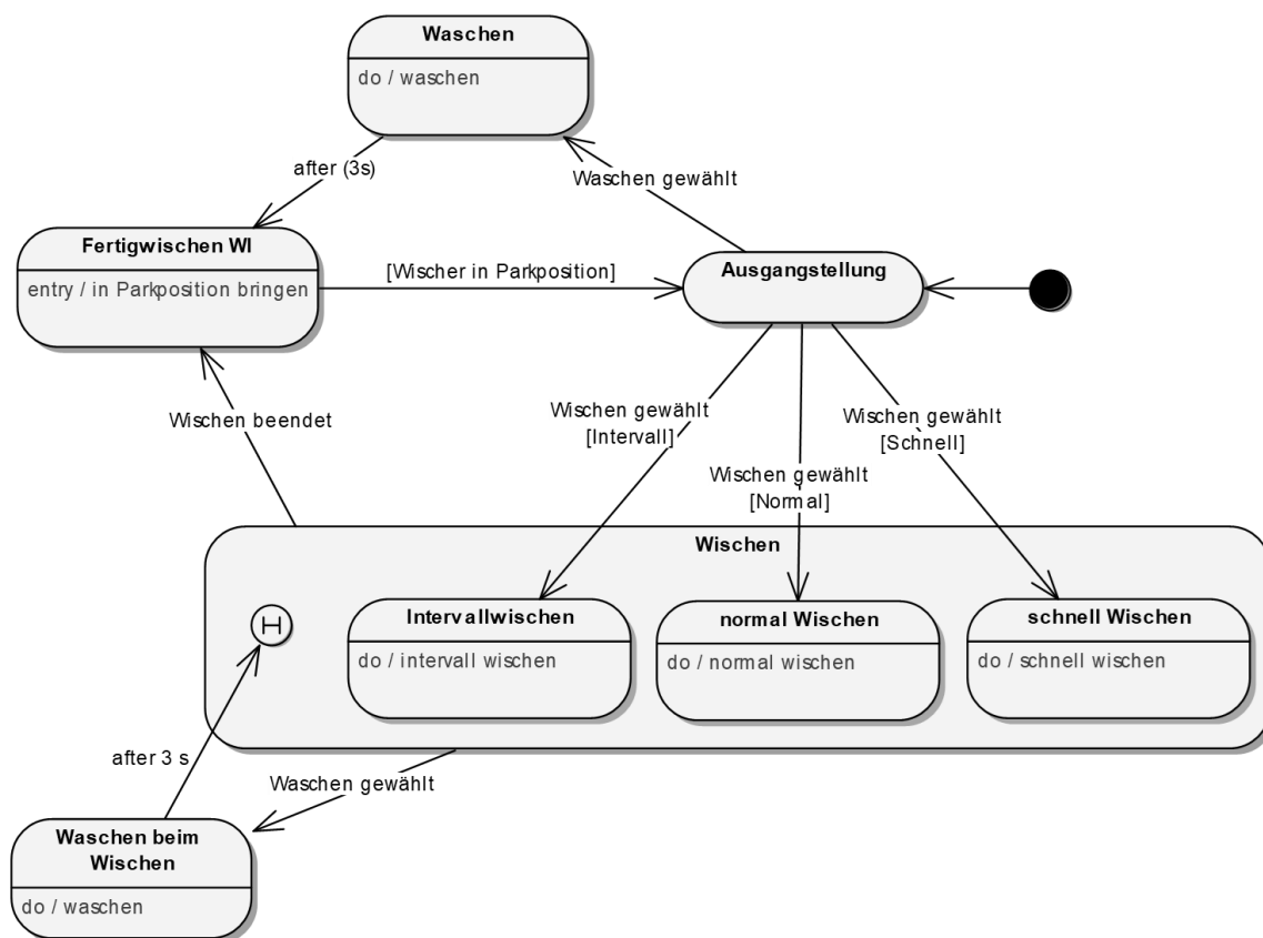
Abbildung 54: Zustandsdiagramm für ein Scheibenwischersystem
