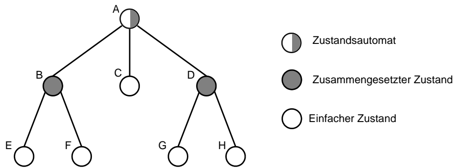
Abbildung 63: Hierarchische Zustände
