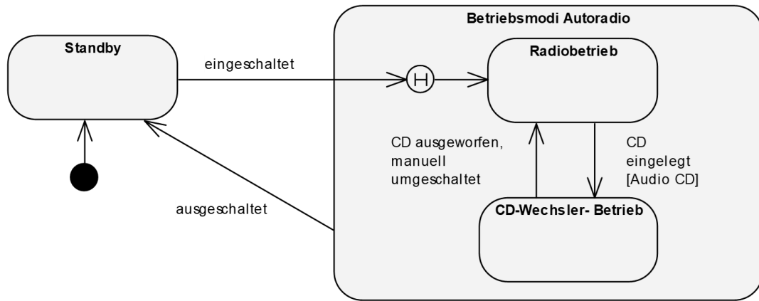
Abbildung 65: Flache Historie
